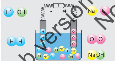
شکل 16.4 میٹل ہیلانڈز کے ڈائلایٹ سلوشنز کی الیکٹرولیسز
